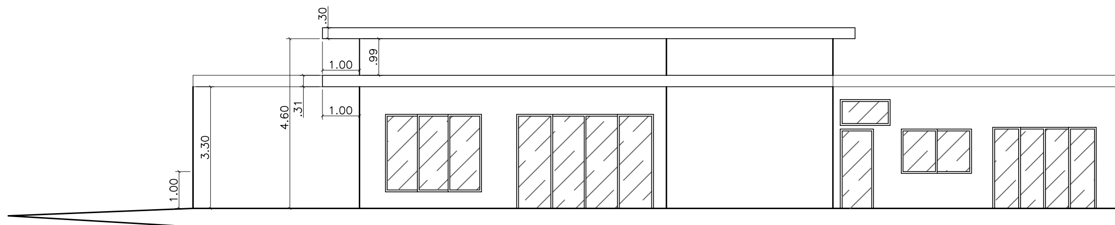
FACHADA AV. 03 - TR. 02 ESCALA 1:100
