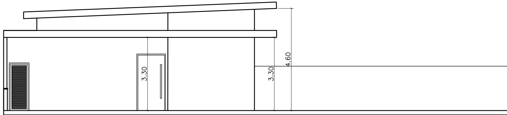
FACHADA RUA APARECIDA DE FREITAS PINTO ESCALA 1:100
